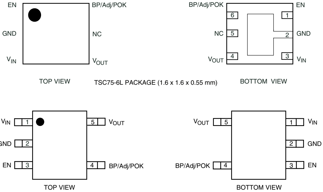
TSOT23-5L/SC70-5L Package
